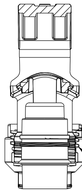
SECTION D-D
